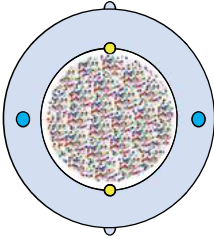
2000心ケーブル (外径23mm)
