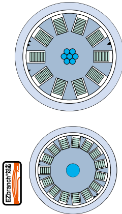
300心型 4心テープ心線タイプ
