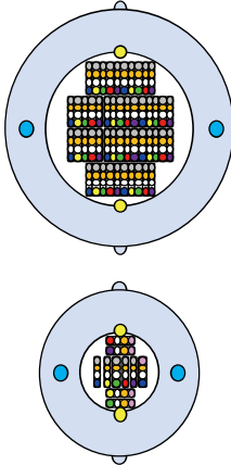
40心型 間欠接合型4心テープ心線タイプ
