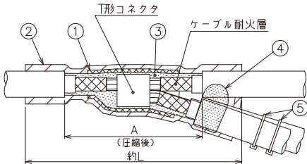
※図面は1相分のみの表示です
