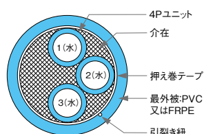
■構造図
