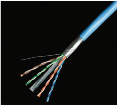
■構造図
