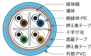
■構造図
