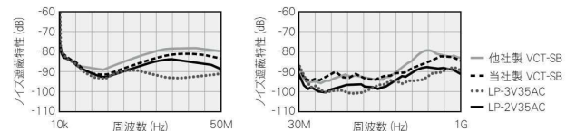
シールド付き電源ケーブルノイズ遮蔽特性
