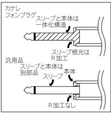
〈フォンプラグ断面〉
