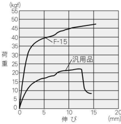
フォンプラグの本体強度試験
