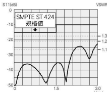
DCP-C25HDのリターンロス
