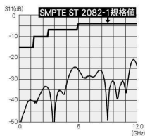
BCJ-D25HWのリターンロス
