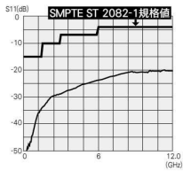
BCP-TKのリターンロス
