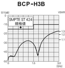
BCP-H3Bのリターンロス
