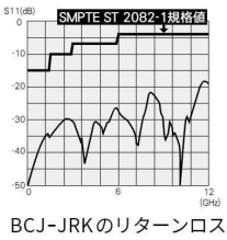
BCJ-JRKのリターンロス
