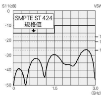
BCP-A3のリターンロス
