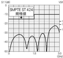
BCP-C6HDのリターンロス
