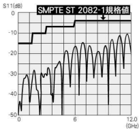
BCP-B5Fのリターンロス
